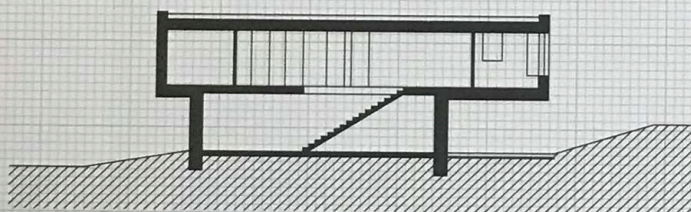
ŘEZ SECTION
